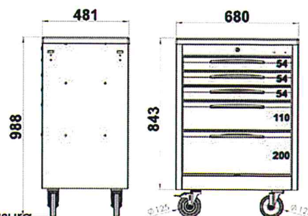
Carrello porta utensili a 5 cassetti mod. FG 150
