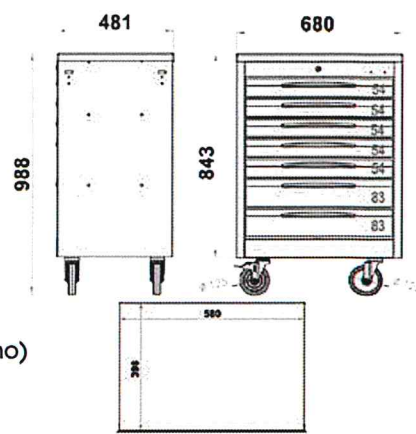
Carrello porta utensili a 7 cassetti mod. FG 103
