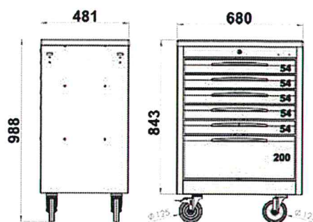
Carrello porta utensili a 6 cassetti mod. FG 150
