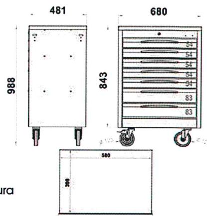
Carrello porta utensili a 7 cassetti mod. FG 150
