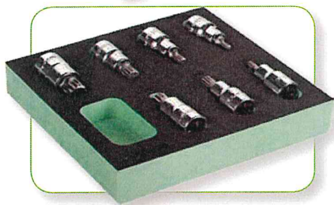
Modulo inserti a bussola da 1/2" con impronta XZN
