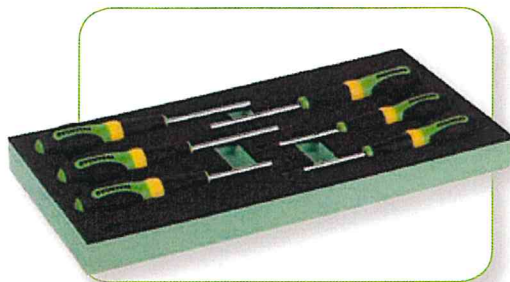
Modulo 6 giraviti ESTRO per viti con impronta TORX
