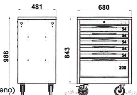
Carrello porta utensili a 6 cassetti mod. FG 103
