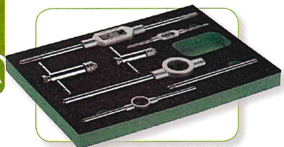
Modulo accessori per maschi a mano e filere
