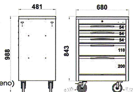
Carrello porta utensili a 5 cassetti mod. FG 103
