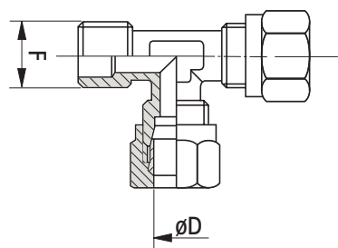
RACCORDO A OGIVA A T LATERALE
