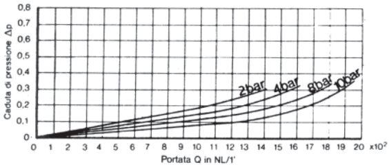
LUBRIFICATORE
