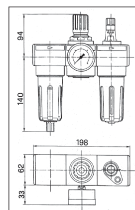
FRL 60 GRUPPO COMPLETO A TRE ELEMENTI
