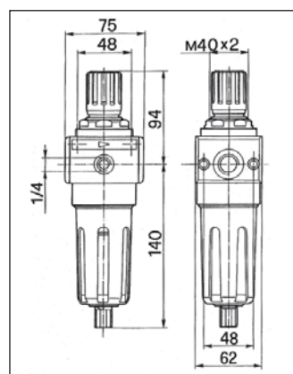
FR60 TM FILTRO-REGOLATORE DI PRESSIONE 42141833
