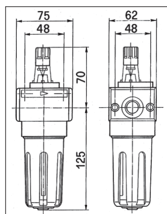
L60 TM LUBRIFICATORE A MICRONEBBIA 42121663
