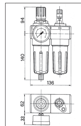
FR+L 60 GRUPPO COMPLETO A DUE ELEMENTI
