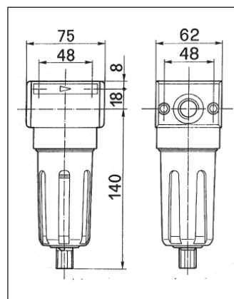
F60 TM FILTRO SEPARATORE DI CONDENZA 42111813
