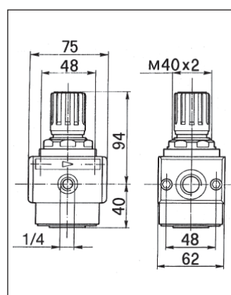
R60 REGOLATORE DI PRESSIONE 42131663
